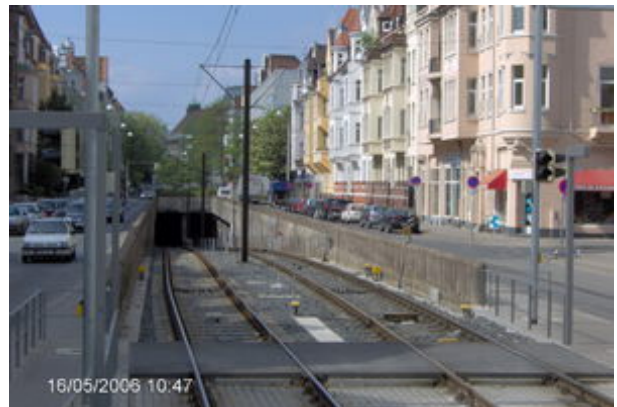
Rampe Hammersteinstraße mit Gleis auf Betonschwelle
